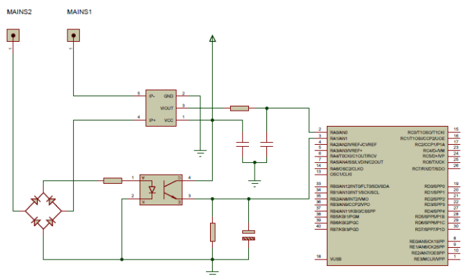
Fig. 5 Watt Meter
